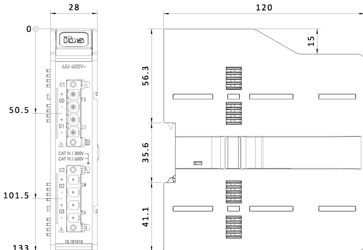
Abmessungen ibaM-4AI-600V-AC , Maße in mm
