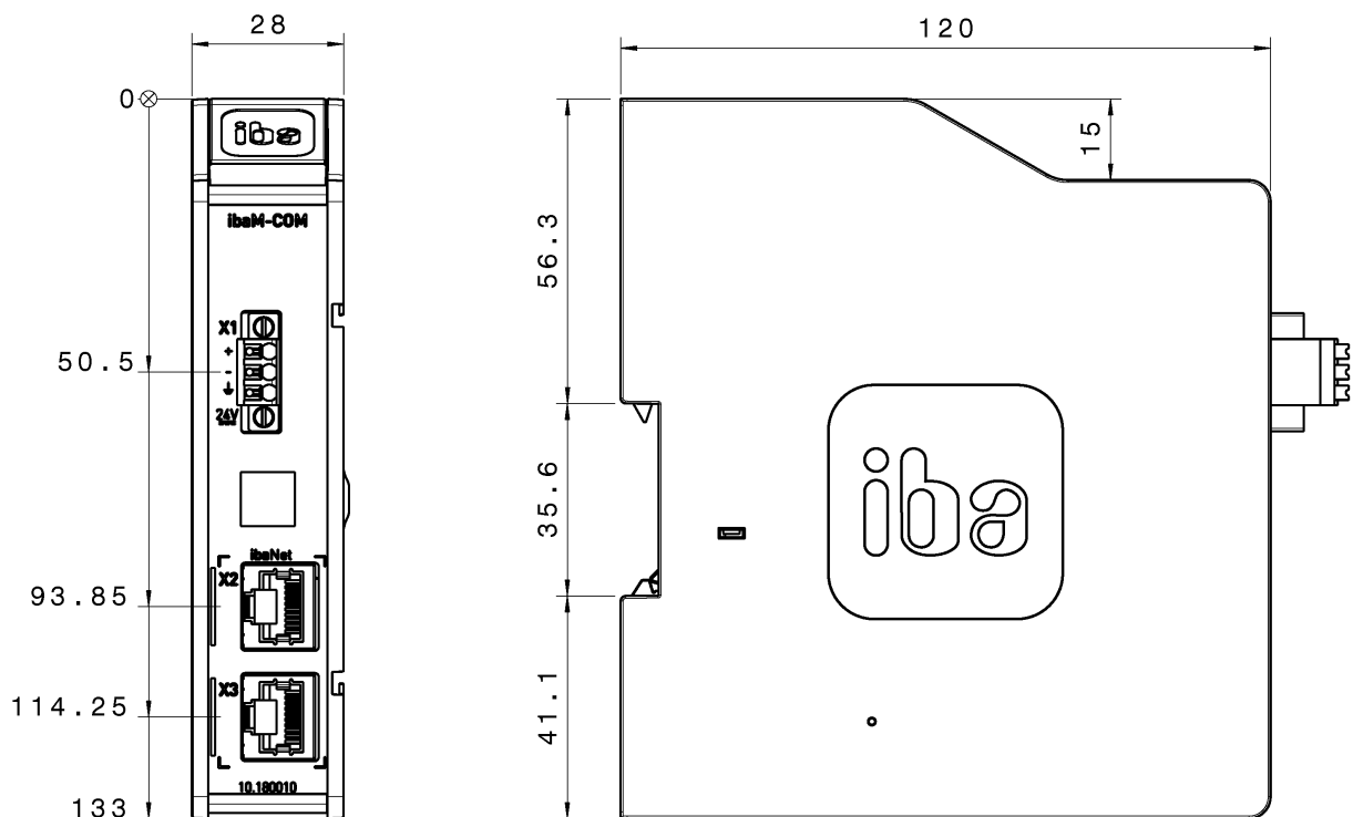
Abmessungen ibaM-COM , Maße in mm
