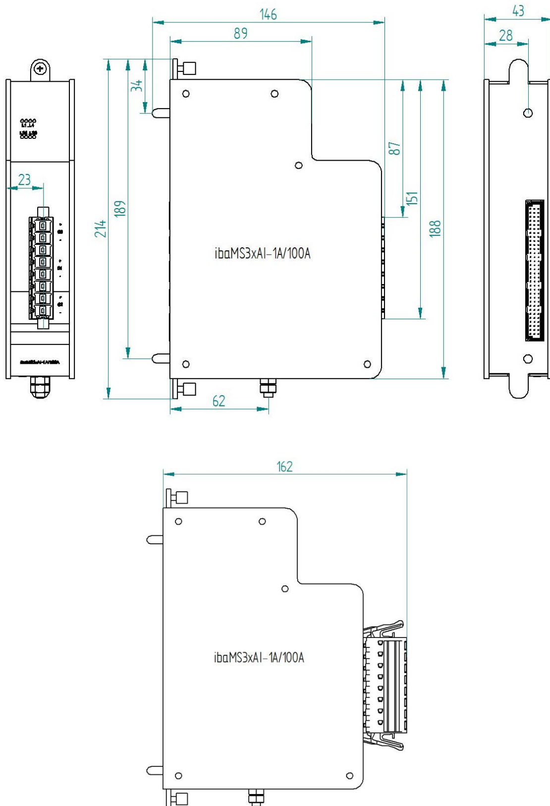
Abmessungen der Module mit Steckverbinder (Maße in mm)
